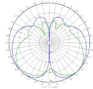
指向性特性例(垂直面) 青色:90MHz 緑色:215MHz
