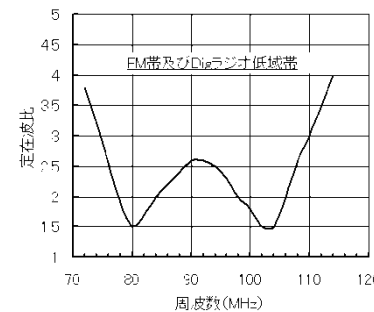
VSWR(参考計算値)
