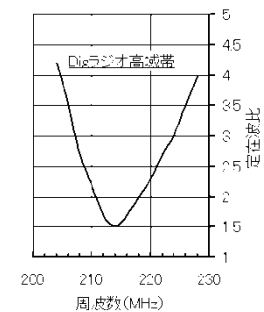
VSWR(参考計算値)
