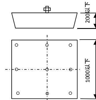
外観図
