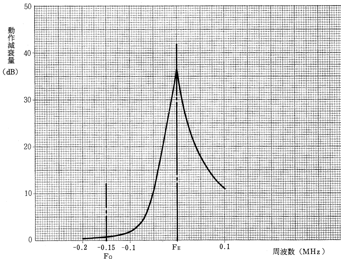
減衰特性例
