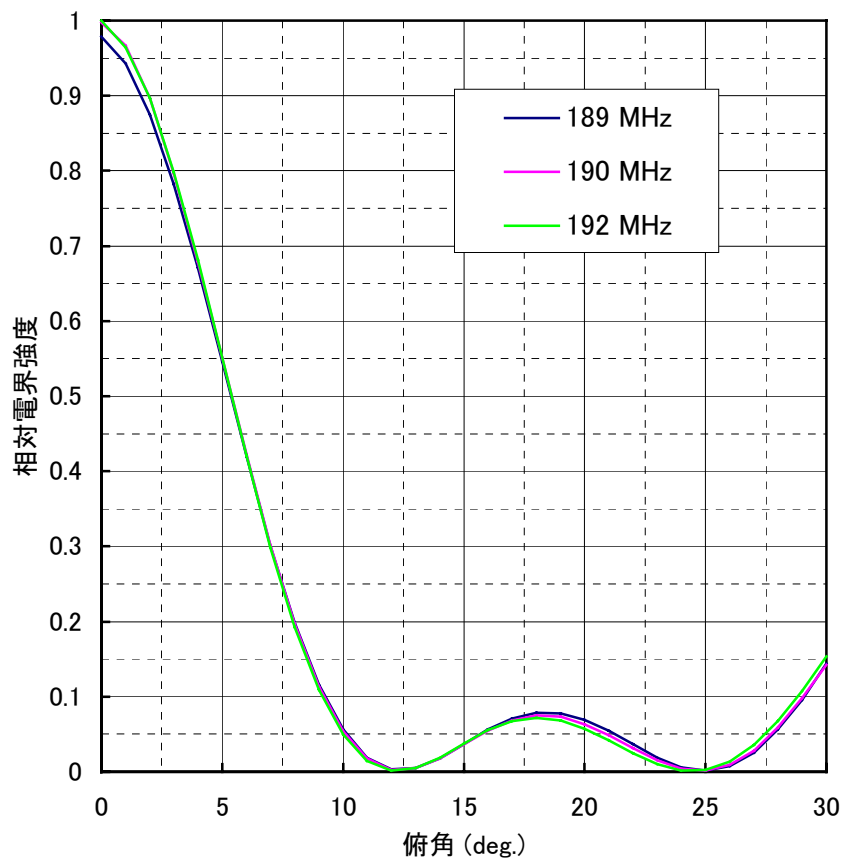
垂直面内指向性
